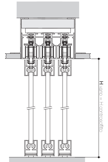
VISTA IN SEZIONE
