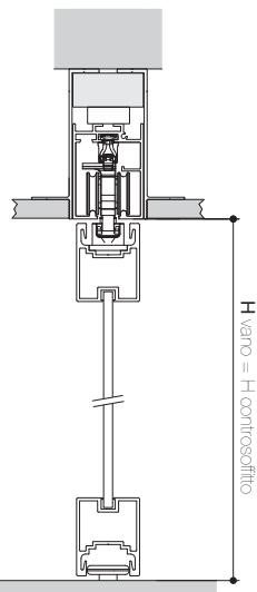
VISTA IN SEZIONE
