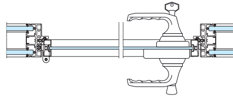
PORTA BATTENTE TUTTO VETRO
