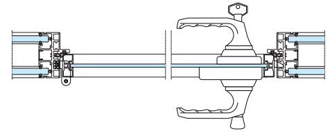
PORTA BATTENTE A PANNELLO MELAMINICO
