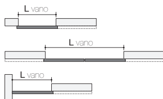
VISTA IN PIANTA
