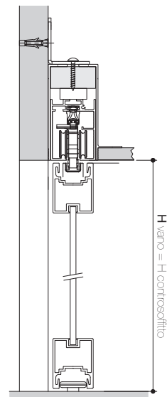
VISTA IN SEZIONE
