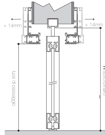
VISTA IN SEZIONE
