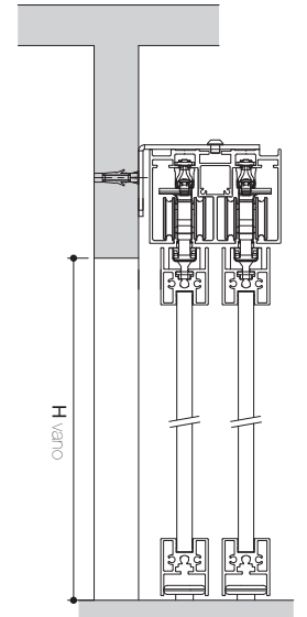
VISTA IN SEZIONE
