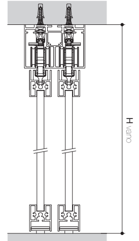
VISTA IN SEZIONE
