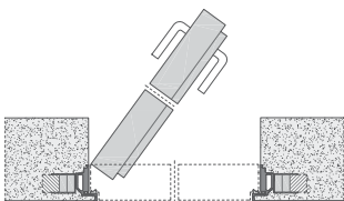
MURATURA SPINTA SINISTRA
