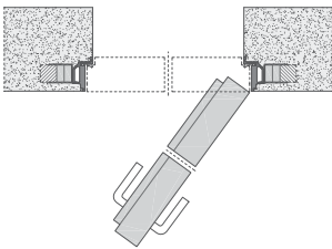
MURATURA TIRA SINISTRA
