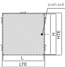
TELAIO 3 LATI ANTA SINGOLA
