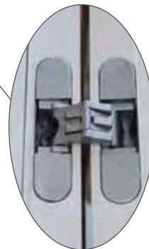
Per mimetizzare la cerniera metallica viene applicata una cover sagomata ad incastro da montare dopo la pittura.
