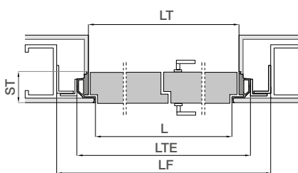
APERTURA A SPINTA
