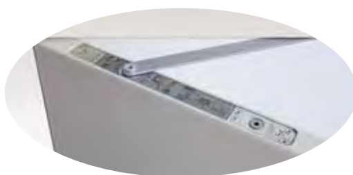
CHIUDIPIORTA AD INCASSO IDEALE PER SERRATURA A RULLO
