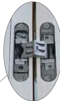
Le cerniere a scomparsa garantiscono la linearità e l'essenzialità del sistema porta, grazie alla tripla regolazione sui tre assi.
