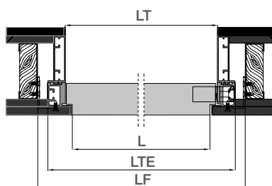
APERTURA A SPINTA
