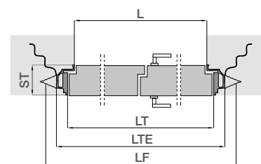
APERTURA A TIRARE
