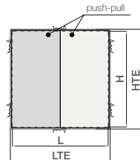
TELAIO 4 LATI ANTA DOPPIA
