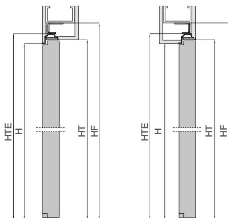
APERTURA A SPINTA
