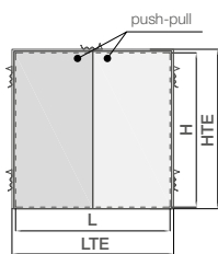
TELAIO 3 LATI ANTA DOPPIA
