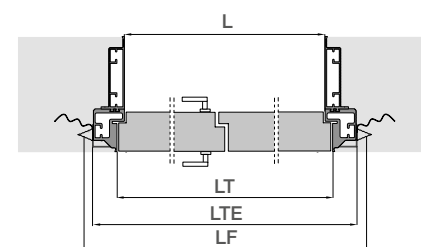
APERTURA A TIRARE
