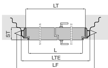
APERTURA A SPINTA
