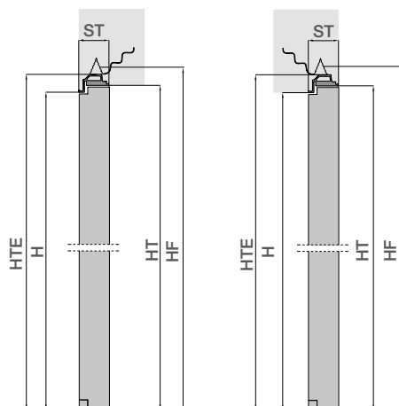
APERTURA A SPINTA
