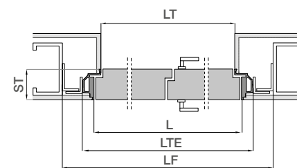
APERTURA A TIRARE
